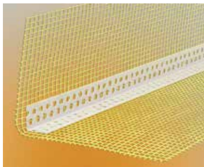
PVC-Eckwinkel mit Gewebe 10 x 15 cm, Länge 2,5 m, weiß, Eckverstärkung an Gebäudeecken und Wandöffnungen
