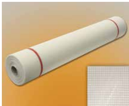
VWS Gewebe weiß 1 x 50 m, 160 g, Maschenweite 4 x 4 mm, hochreißfestes Glasseeidengittergewebe
